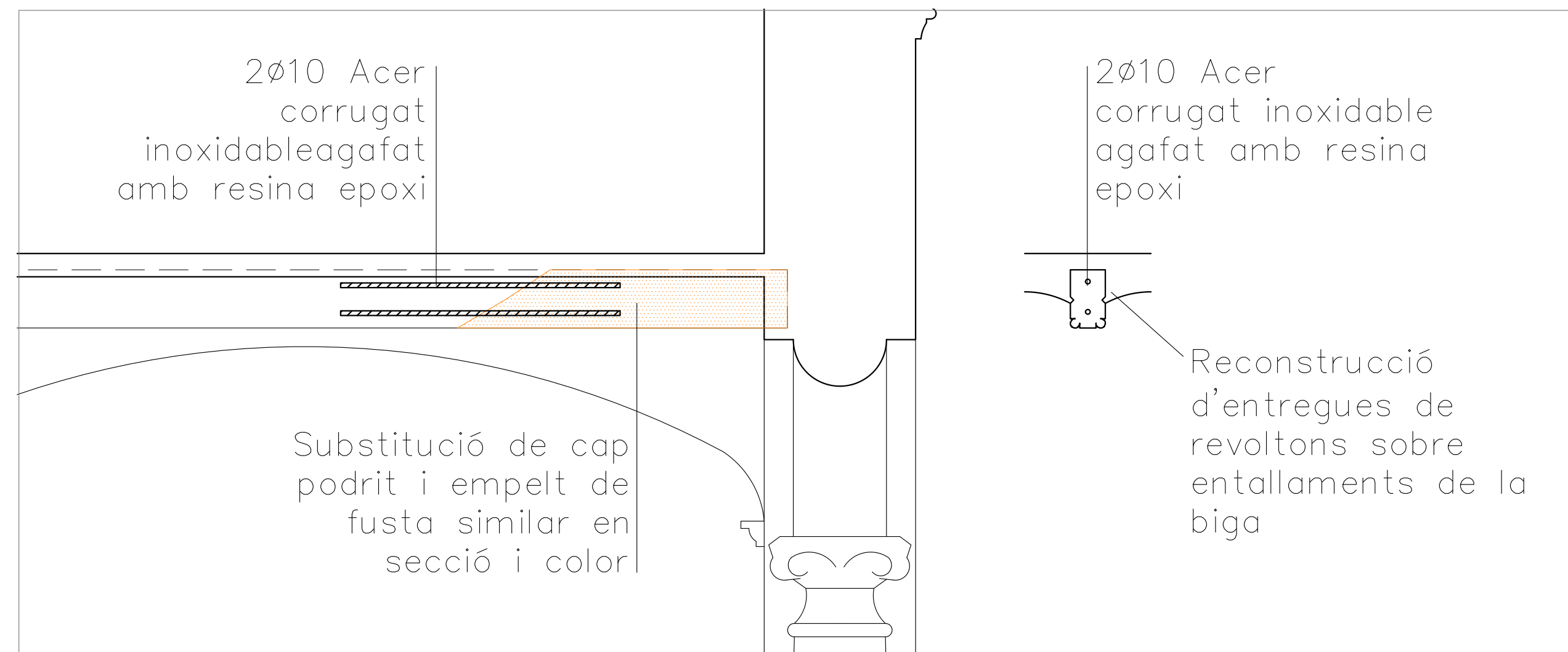
DETALL EMPOLT NOU CAP DE BIGA 1/20
