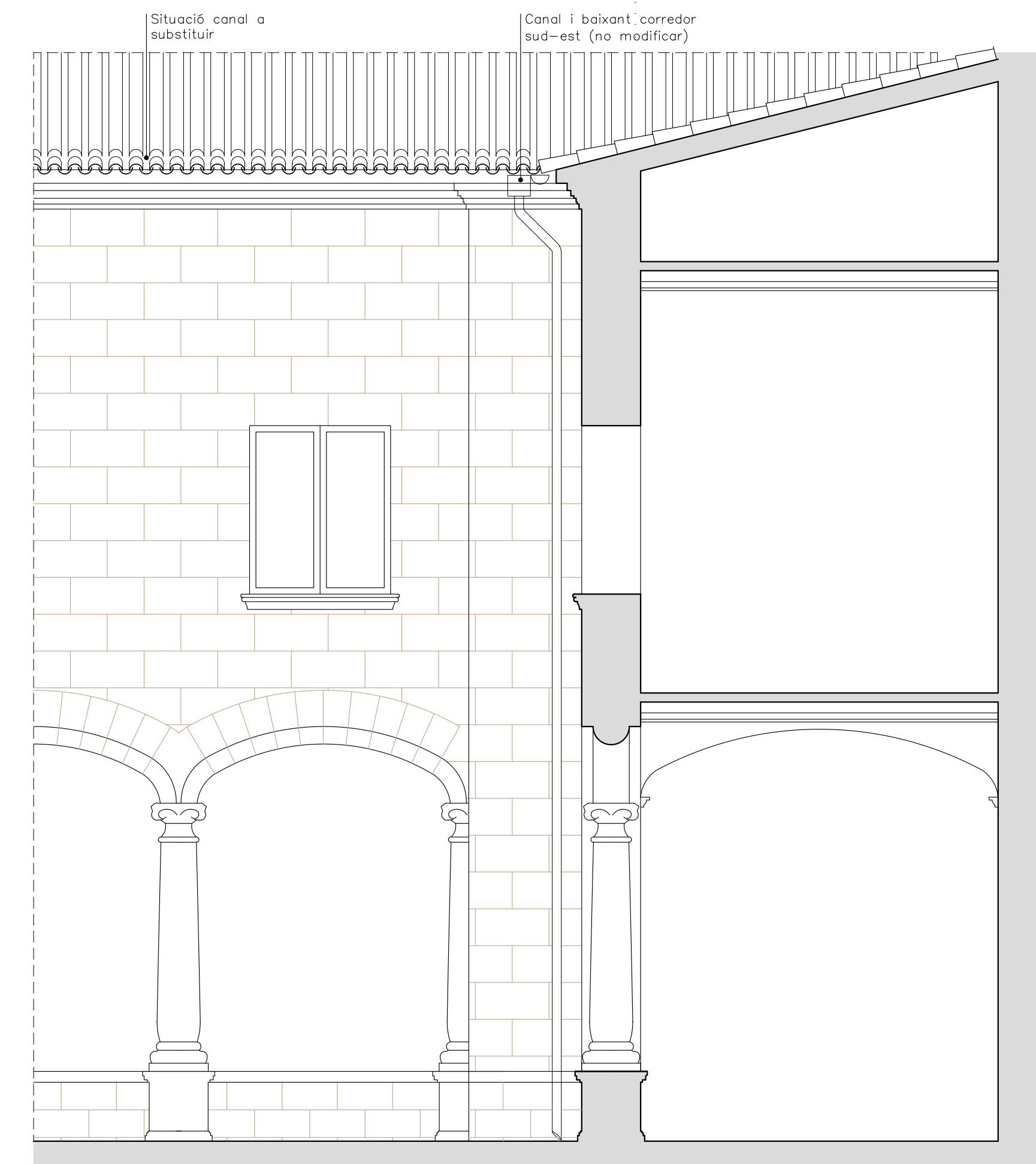
ALÇAT CANTONADA EST
